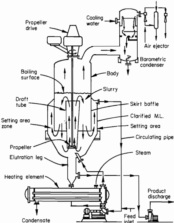
Fig. 9 Draft-tube-baffle (DTB) crystallizer.
